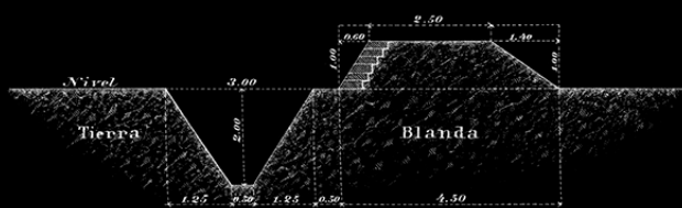
SECCION TRASVERSAL DE LA ZANJA EN TOSCA Y TIERRA
